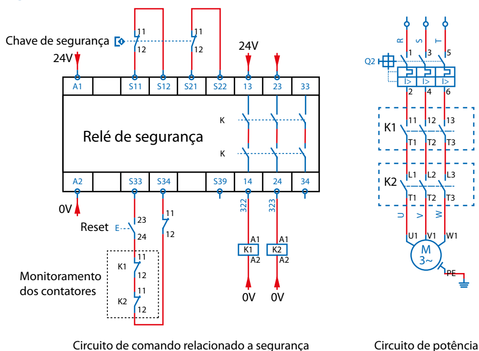
Figura 8 – Exemplo de monitoramento de contator
